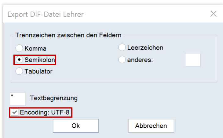
Abbildung 1: Einstellungen für den Export aus Untis.
