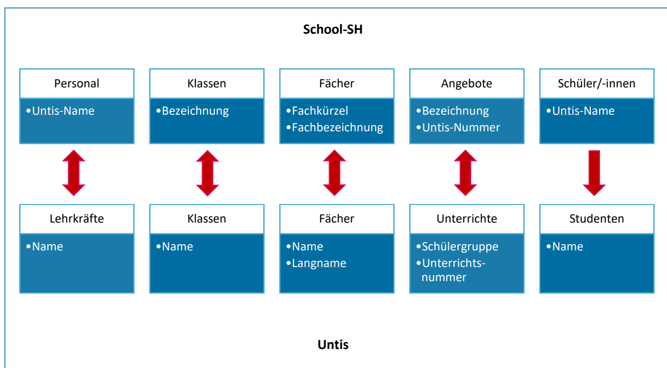
Abbildung 3: Datenbeziehungen zwischen School-SH und Untis
